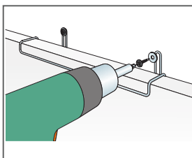
Крепление материала класса A2(нержавеющая сталь) на шуруп
